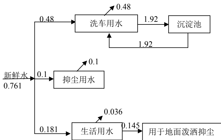
图 2-1 项目水量平衡图 单位：m 3 /d
