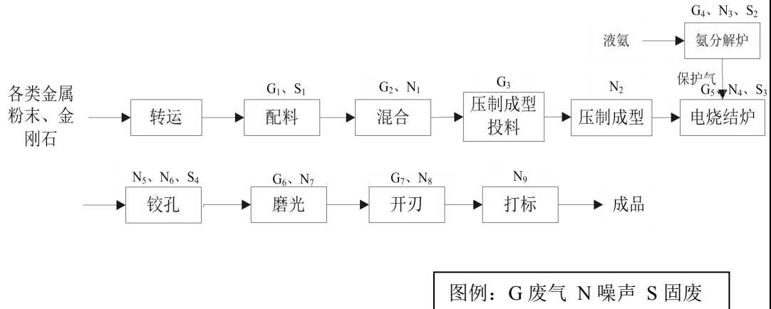
图 2-2 金刚石磨盘工艺流程及产污节点图
