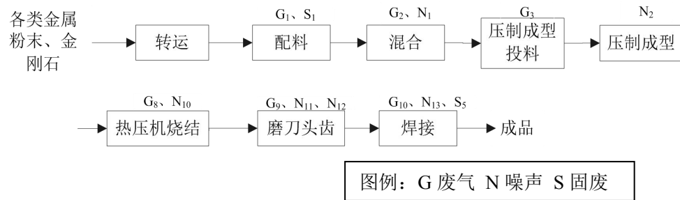
图 2-3 金刚石薄壁水钻工艺流程及产污节点图
